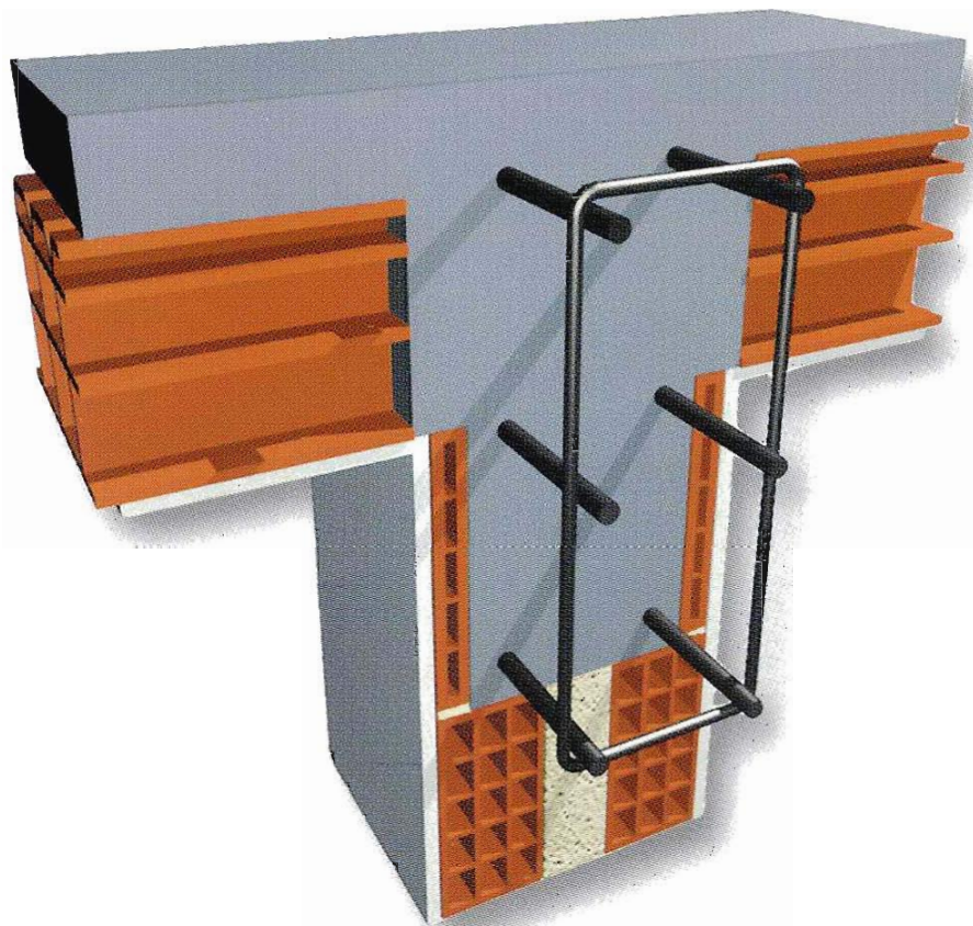
Fig. 33 - Rivestimento di una trave non contenuta nello spessore del solaio con tavelle di laterizio al fine di realizzare un supporto omogeneo sotto l'intonaco.
