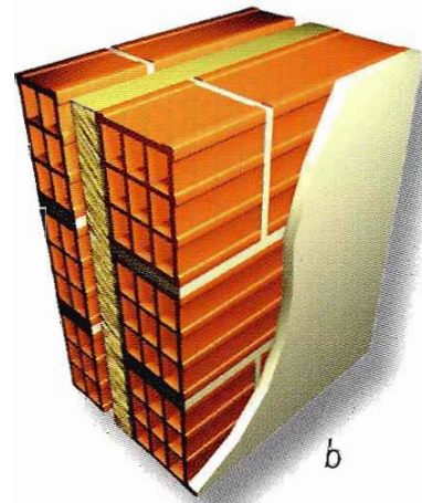
Fig. 3a, b - Pareti doppie per interni, o per tamponamenti esterni, senza e con isolante, con due tavolati di elementi forati di laterizio di uguale o diverso spessore.
