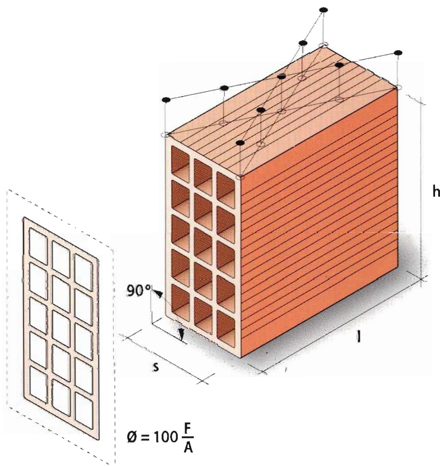
Fig. 6 - Gli elementi forati di laterizio devono rispondere a requisiti di qualificazione e di collaudo che, fra gli altri, riguardano: le dimensioni, la planarità delle facce lungo le diagonali, la rettilineità degli spigoli, la percentuale di foratura ( \emptyset ).
