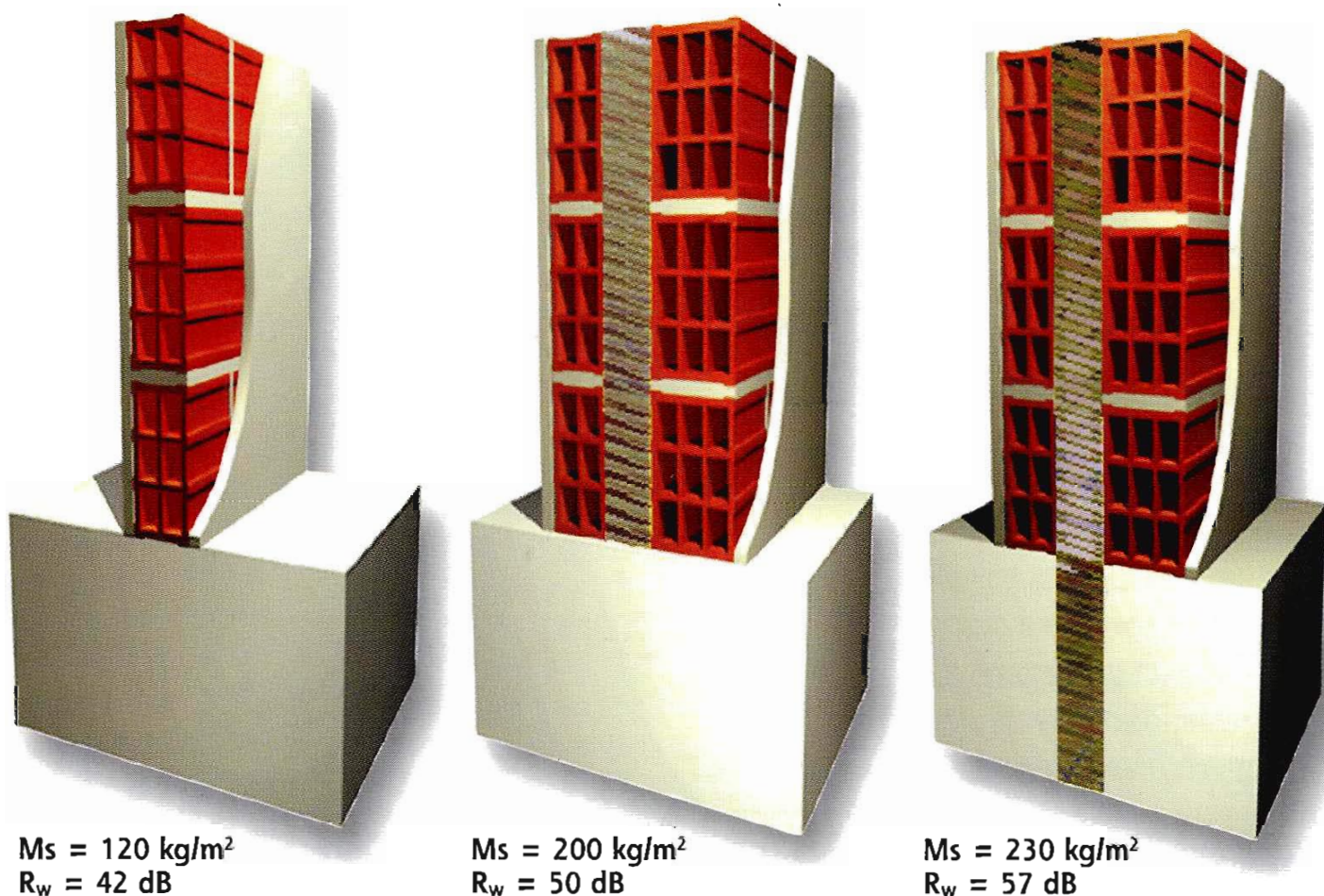
Fig. 25 - Numerose prove di laboratorio permettono di documentare l'indice di valutazione del potere fonoisolante R_w di pareti semplici e doppie in elementi forati di laterizio. Per le pareti doppie i livelli prestazionali sono molto diversi in funzione delle condizioni di integrazione con le strutture perimetrali. Le prestazioni più elevate si ottengono con pareti doppie isolate acusticamente nell'intercapedine e con i due tavolati completamente indipendenti.
