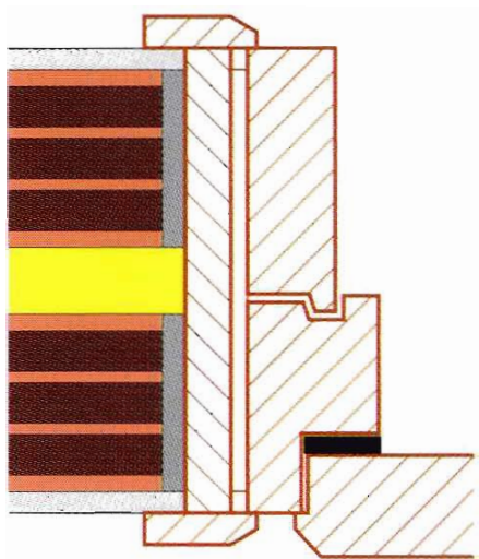
Fig. 39 - Sezione orizzontale di portoncino in legno su parete doppia isolata acusticamente. Si noti la guarnizione acustica alla battuta del portoncino per migliorarne il potere fonoisolante.
