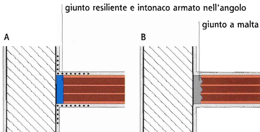
Fig. 32 - Giunto resiliente orizzontale e verticale per parete di ridotto spessore posta in un telaio in cemento armato (per A e B si veda il dettaglio).
