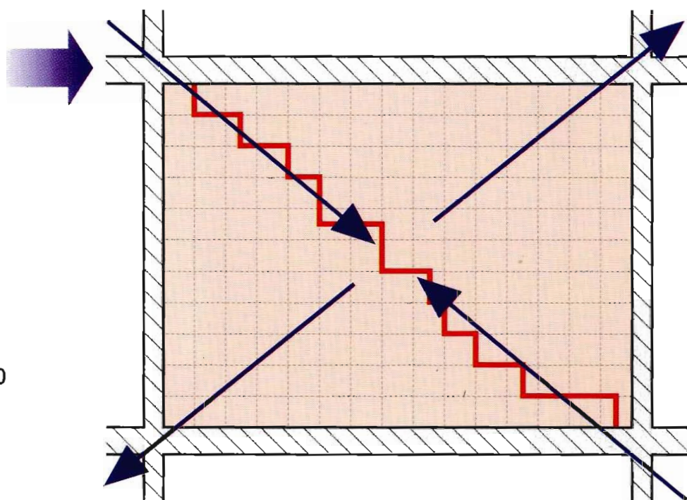
Fig. 21 - Parete rigidamente collegata ad un telaio in cemento armato sottoposto a sollecitazioni orizzontali nel suo piano. Il divisorio contrasta le eventuali deformazioni del telaio, che producono sollecitazioni di compressione e trazione ad andamento diagonale nel divisorio, con conseguenti possibili fessurazioni.
