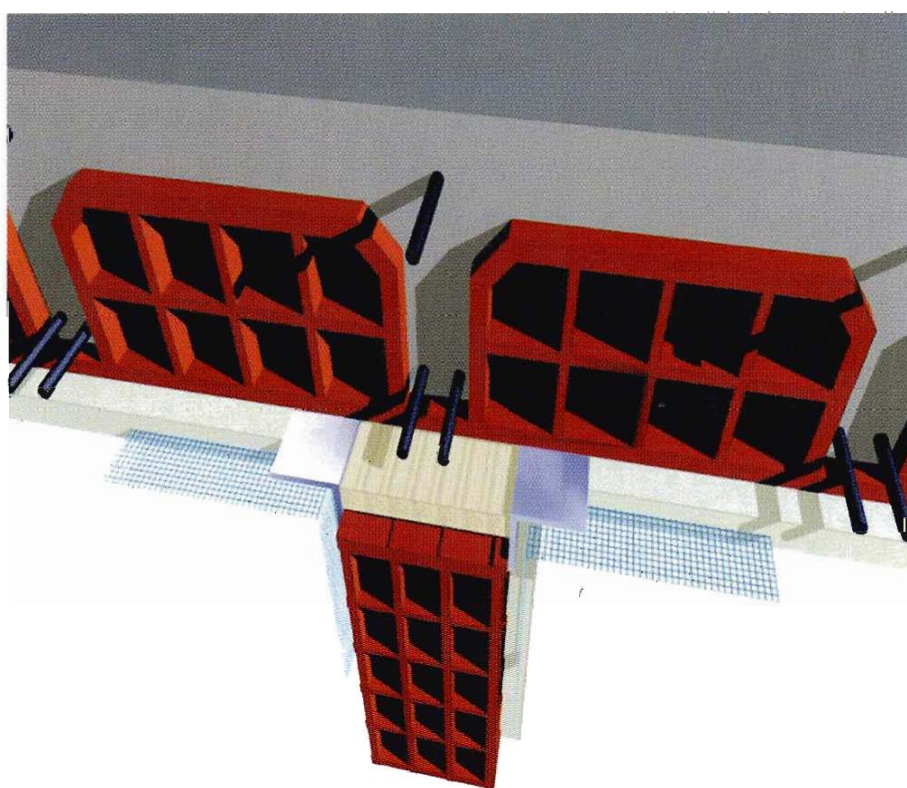
Fig. 30 - Giunto in materiale resiliente fra la parete e l'intradosso del solaio. La striscia resiliente ha uno spessore minimo di 10 mm. Lo spostamento orizzontale della parete è impedito da due angolari posti sotto l'intonaco, eventualmente rinforzato con rete.
