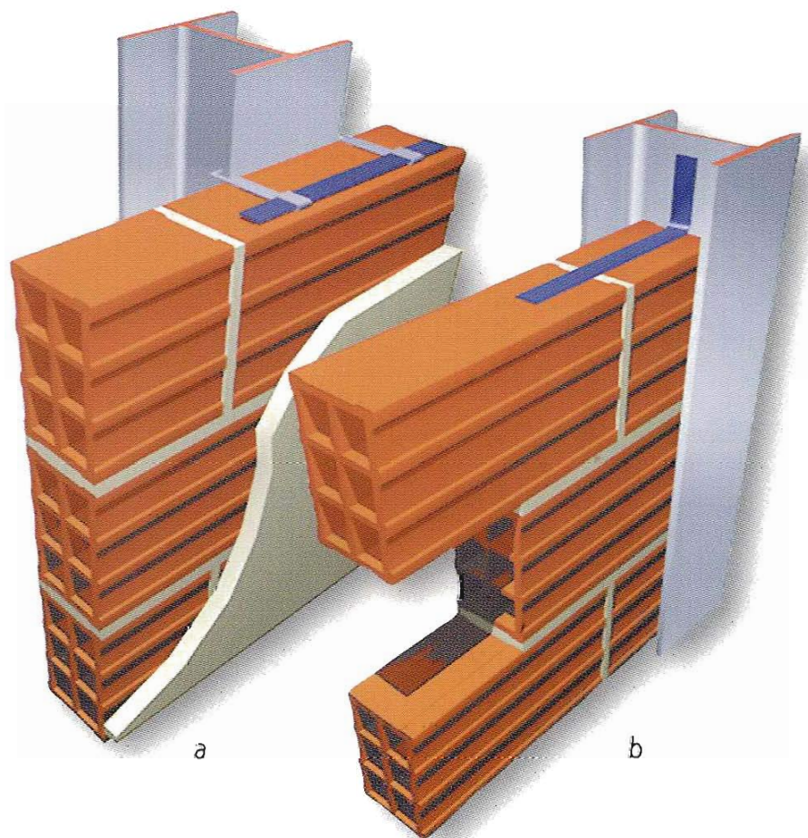
Fig. 34 - Collegamento di una parete in elementi forati di laterizio a un profilato in acciaio mediante staffe poste nei giunti orizzontali: a) parete passante; b) parete inserita.
