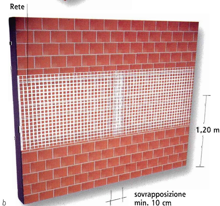
Fig. 14a - Intonaco armato con rete immersa in uno strato di rasante collante (spessore 2 \div 5 mm secondo il tipo di rete).
