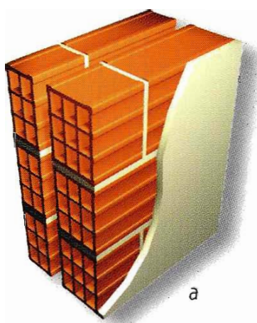
Fig. 3a, b - Pareti doppie per interni, o per tamponamenti esterni, senza e con isolante, con due tavolati di elementi forati di laterizio di uguale o diverso spessore.
