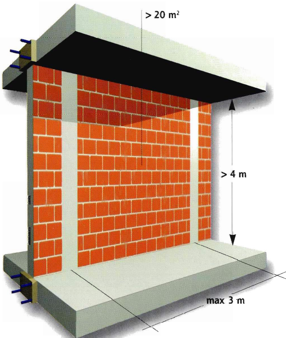
Fig. 22 - In zona sismica, nel caso di parete divisoria di grandi dimensioni, sono da prevedere collegamenti al telaio in cemento armato, con irrigidimenti ad interasse non superiore a 3 metri.
