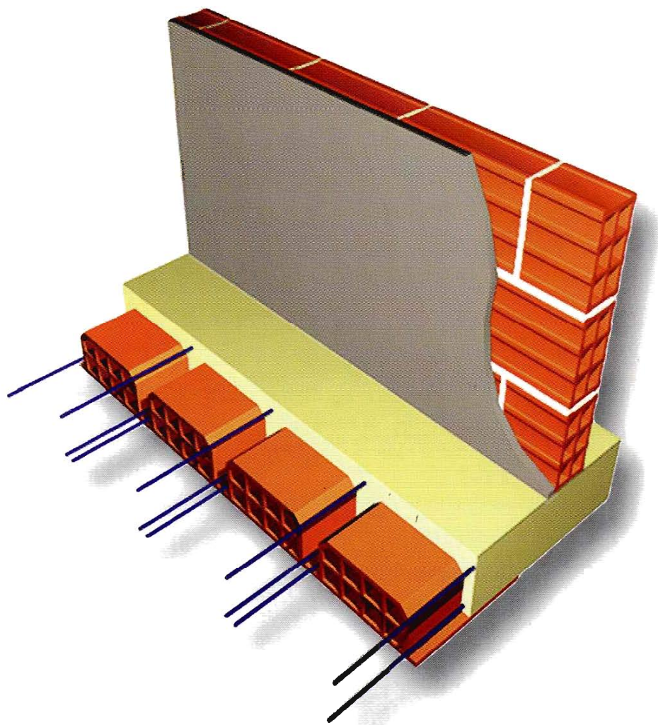
Fig. 16 - Parete divisoria disposta trasversalmente alle nervature del solaio.
