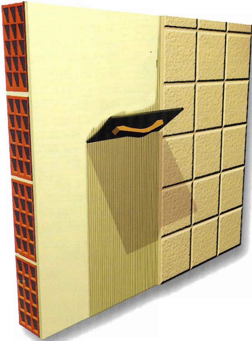
g. 15 - Rivestimento ceramico posato con adesivo cementizio, steso sulla parete con spatola dentata, dopo l'intonacatura e la preparazione con una mano d'imprimitura.
