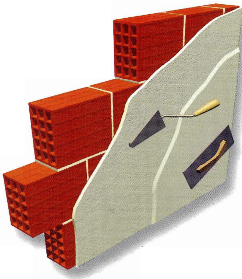
Fig. 13 - L'intonaco tradizionale si stende a mano. Il primo strato è gettato con la cazzuola contro la parete; lo strato di finitura viene lisciato con cazzuola metallica (finitura a gesso scagliola) o con fratazzo (finitura grezza) o con fratazzino (finitura liscia). Per ottenere particolari effetti la superficie lisciata può essere spazzolata con spazzola metallica.
