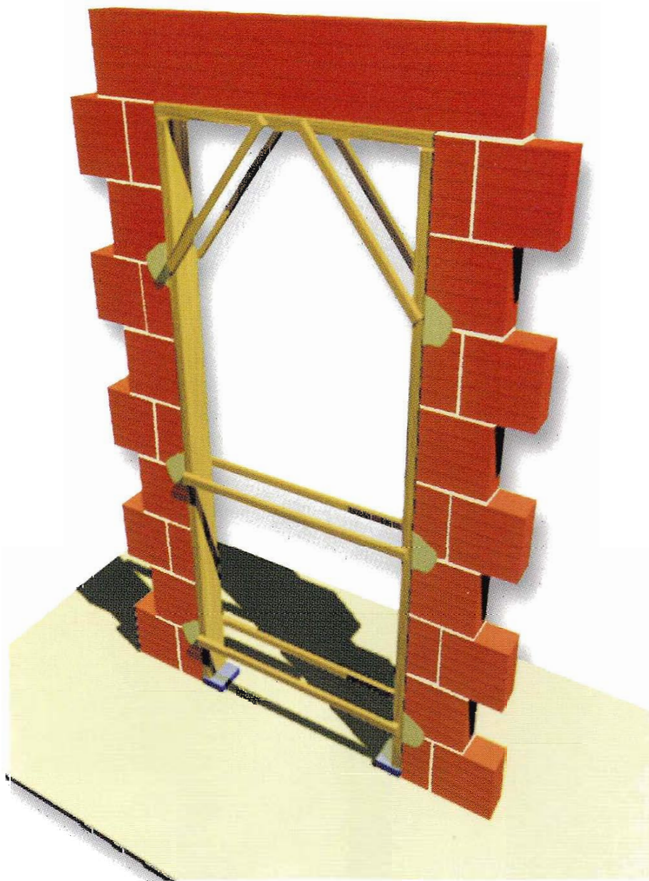
Fig. 37 - Realizzazione del vano porta con architrave in tavellone di laterizio. Montaggio del controtelaio tramite zanche. Si notino i distanziatori alla base del controtelaio in corrispondenza dello spessore del massetto di pavimentazione.
