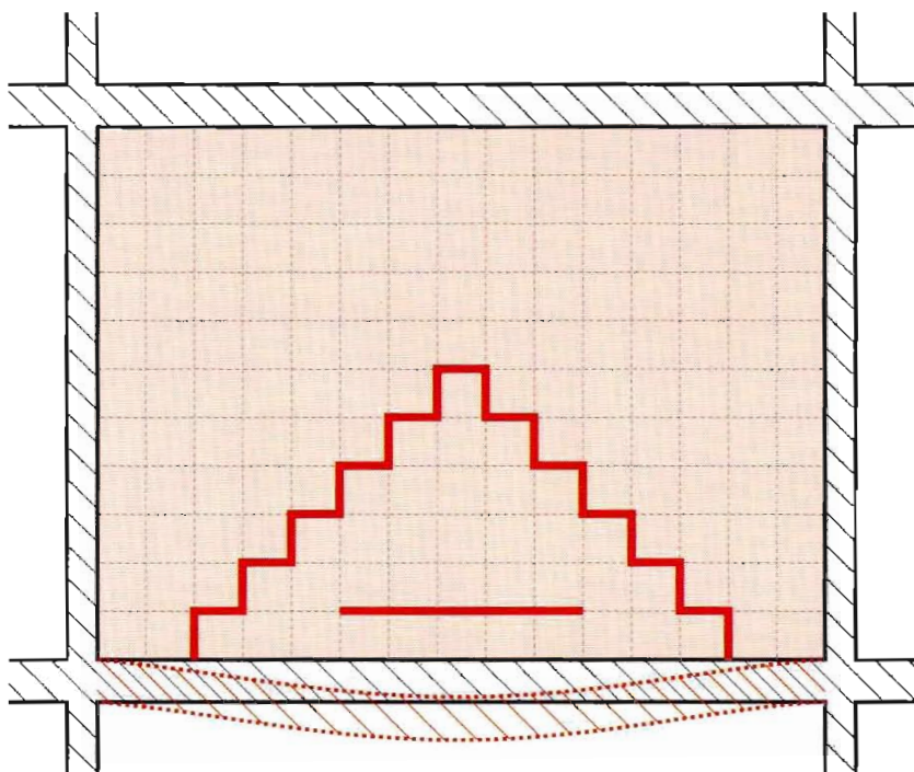
Fig. 19 - Se il solaio inferiore si deforma più di quello superiore la parete divisoria tenderà a fessurarsi con andamenti delle fessure (ad arco o rettilinee secondo la dimensione degli elementi) che denunciano il distacco della porzione di muratura non più sufficientemente supportata.
