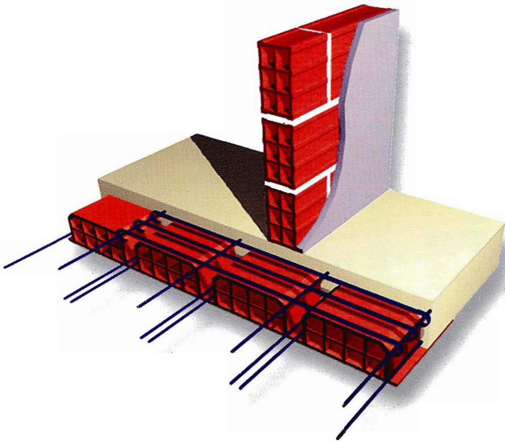
Fig. 17 - In presenza di divisori semplici abbastanza pesanti o di divisori doppi disposti parallelamente ai travetti del solaio, è opportuno rinforzare la struttura con armature trasversali che ripartiscano il carico su più nervature.
