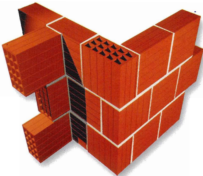
Fig. 35 - Formazione di un angolo e di un innesto a T fra pareti in elementi forati di laterizio.
