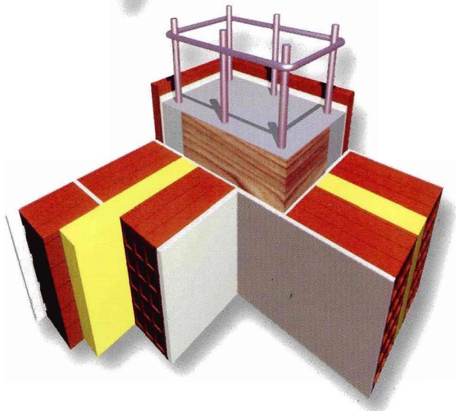
Figg. 48-49 - Giunti di parete esterna doppia in elementi forati di laterizio con pilastri in cemento armato rivestiti da tavole esternamente e da sughero verso l'interno.
