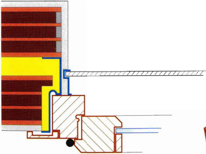
Fig. 47 - Giunto orizzontale con l'infisso di una parete esterna doppia in elementi forati di laterizio, realizzato tramite controtelaio metallico e schiuma isolante interposta. Si noti come il ponte termico sia notevolmente ridotto.
