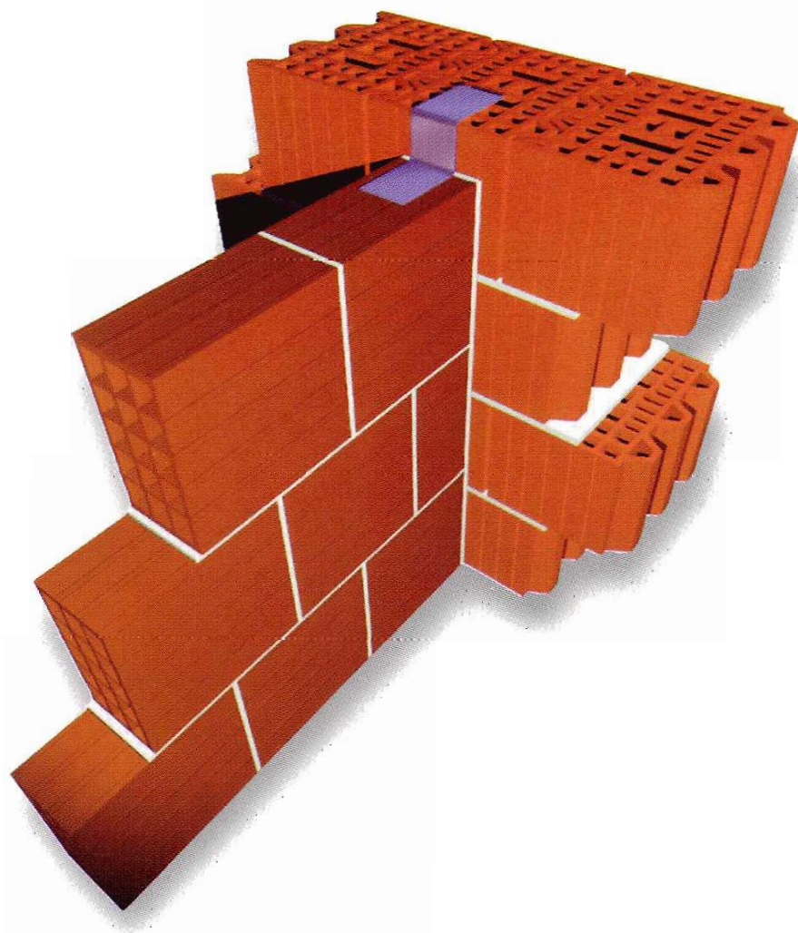
Fig. 36 - Innesto a T fra parete in elementi forati e parete in blocchi a fori verticali, tramite staffa metallica adattabile.
