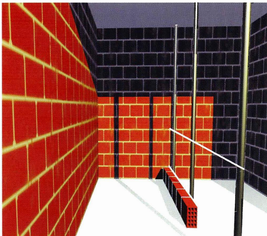
Fig. 29 - Per il tracciamento della posizione della muratura si tende un filo, spostabile in altezza, fra delle aste poste in verticale, a segnare uno dei bordi della parete. Il filo viene progressivamente alzato a segnare il piano di livello per l'allineamento dei corsi.
