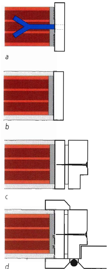
Fig. 38 - Sequenza di montaggio di una porta:
