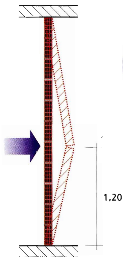
Fig. 20 - Parete sollecitata a flessione in presenza di carico orizzontale perpendicolare al piano della parete.
