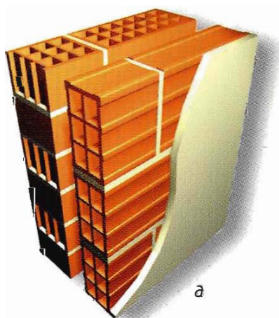
Fig. 4a, b - Pareti doppie per tamponamenti esterni con il tavolato interno in elementi forati, senza e con isolante.
