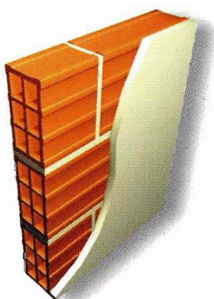
Fig. 2 - Parete semplice per la realizzazione dei divisori interni.
