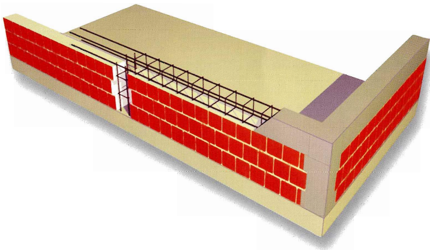
Fig. 46 - Irrigidimenti in cemento armato, opportunamente ammorsati, in un parapetto in elementi forati di laterizio.
