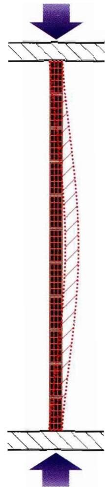
Fig. 18 - Parete sollecitata a flessione in presenza di solaio deformabile.
