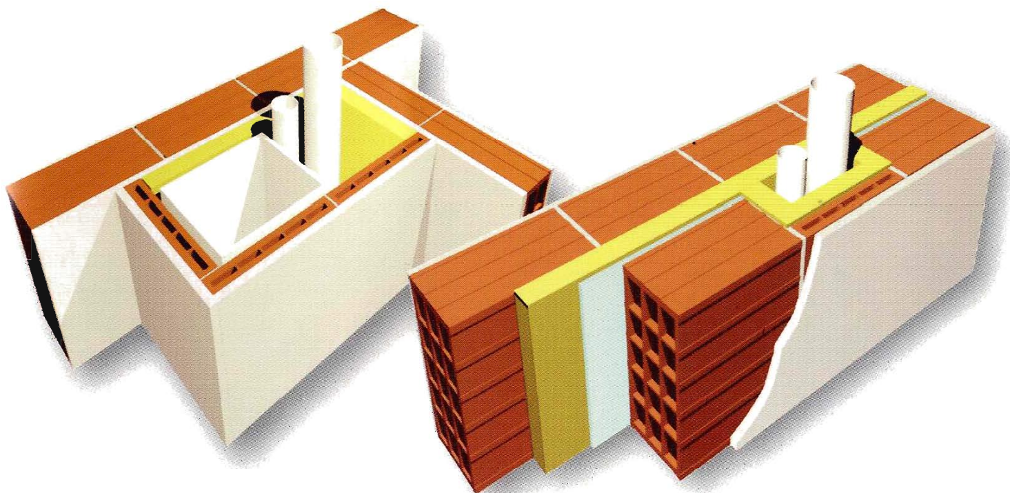
Fig. 44 - Realizzazione di un cavedio con tavole di laterizio e isolamento acustico all'interno.
