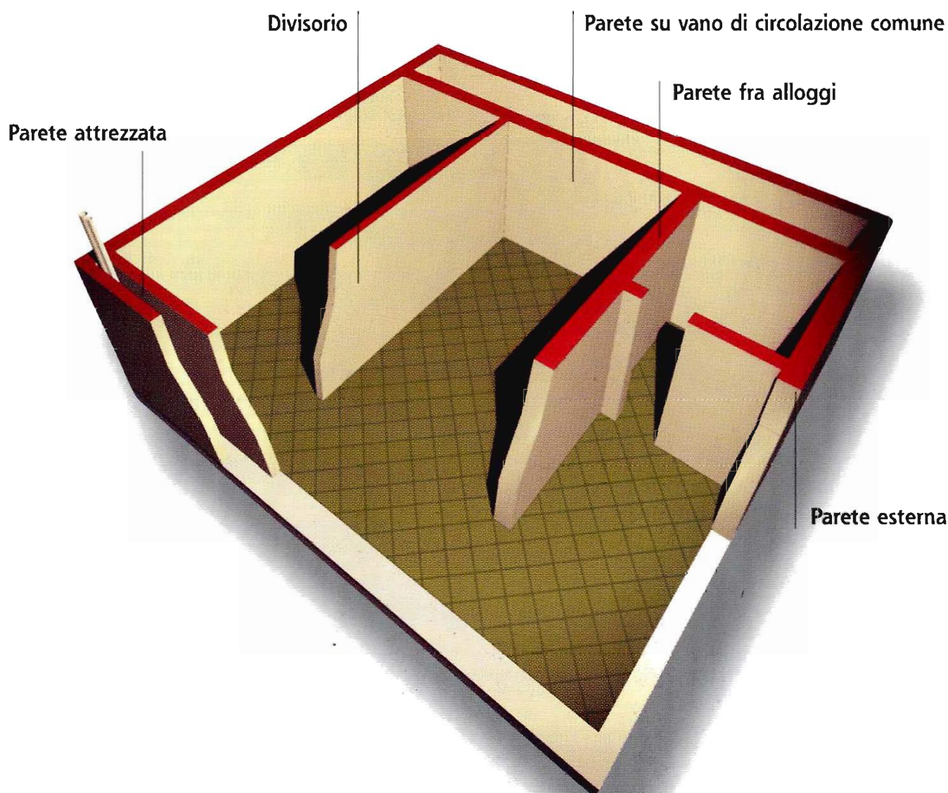
Fig. 1 - Possibili funzioni delle pareti in elementi forati di laterizio.
