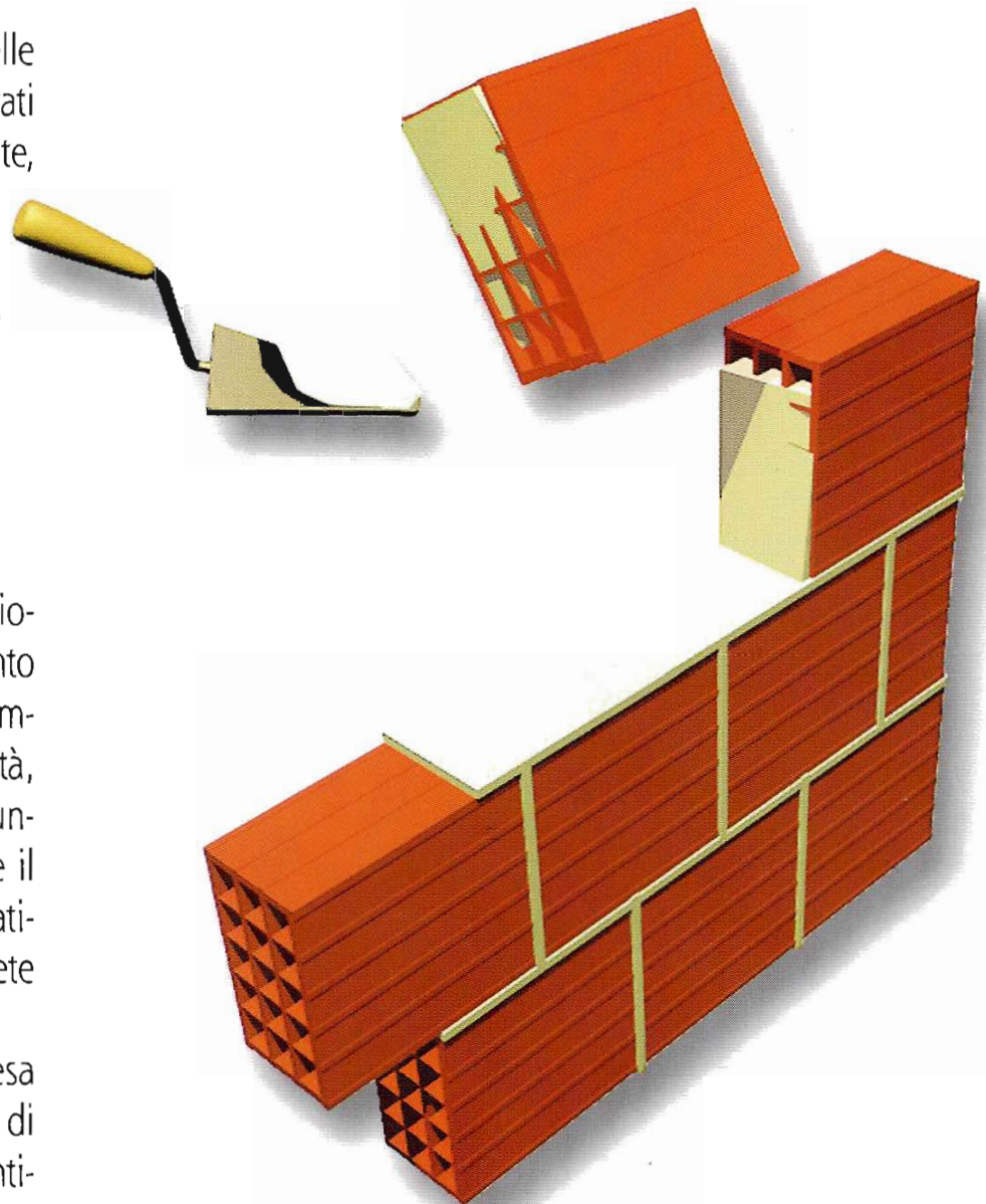
Fig. 11 - Giunti orizzontali e verticali fra gli elementi completamente riempiti a malta.
