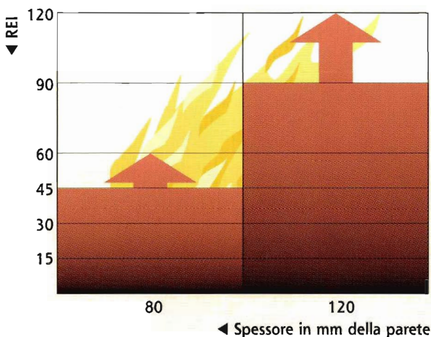
Fig. 28 - Resistenza al fuoco REI di pareti intonacate in elementi forati di laterizio di spessore pari a 8 e 12 cm escluso l'intonaco.
