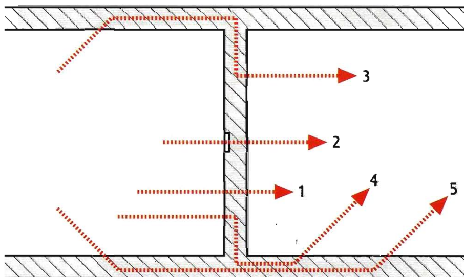
Fig. 24 - La trasmissione sonora fra due ambienti interni dipende dalla trasmissione diretta attraverso la parete di separazione (1), da eventuali trasmissioni dovute alla presenza di condotti di ventilazione, cavedi, reti di impianti ecc. (2) e dalla trasmissione dovuta al contributo delle strutture laterali degli ambienti interni (3, 4, 5). Il potere fonoisolante ( R ) di una parete è riferito alla trasmissione sonora tipo 1, il potere fonoisolante apparente ( R' ) alle trasmissioni sonore tipo 1,3,4,5.
