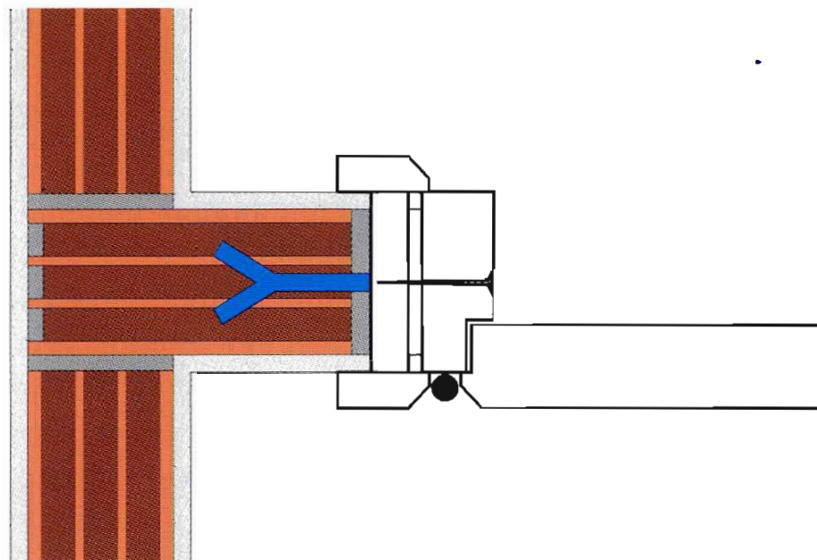
Fig. 40 - Sezione orizzontale della soluzione di montaggio di una porta in prossimità di un angolo.
