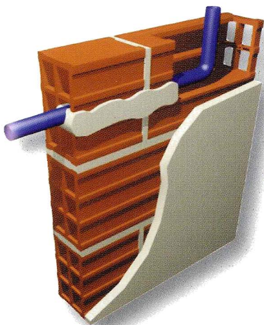
Fig. 42 - Chiusura a malta delle tracce prima dell'intonacatura.
