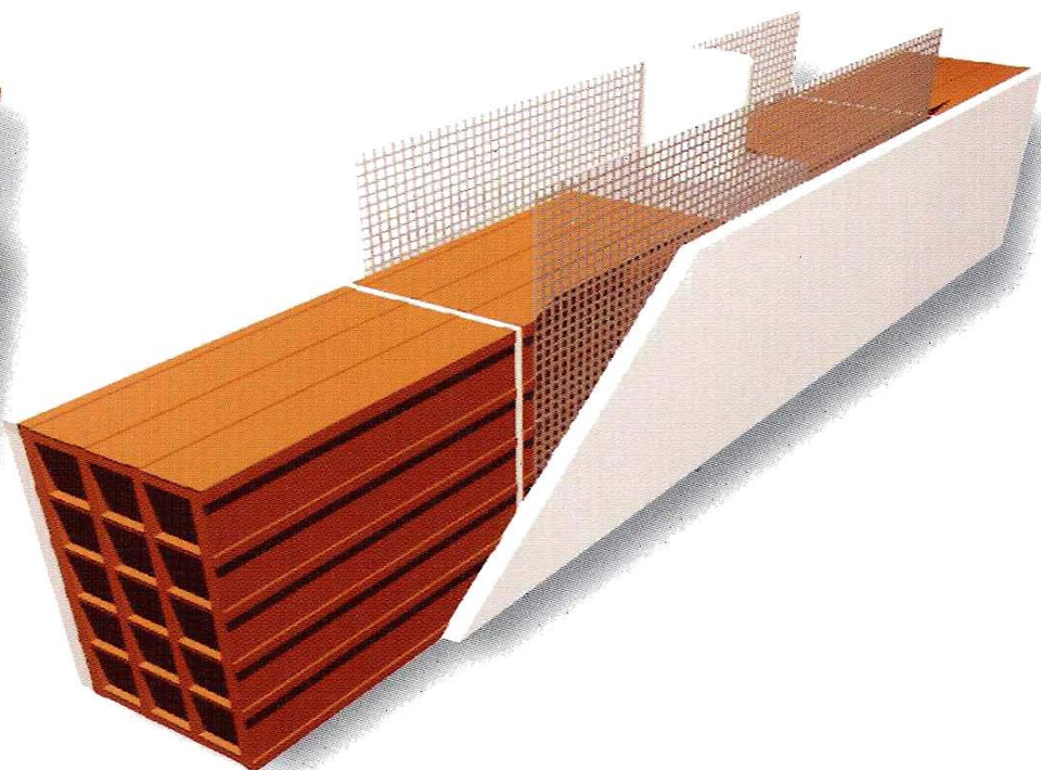
Fig. 43 - Incasso di una tubazione isolata acusticamente, con riempimento in calcestruzzo e armatura dell'intonaco.
