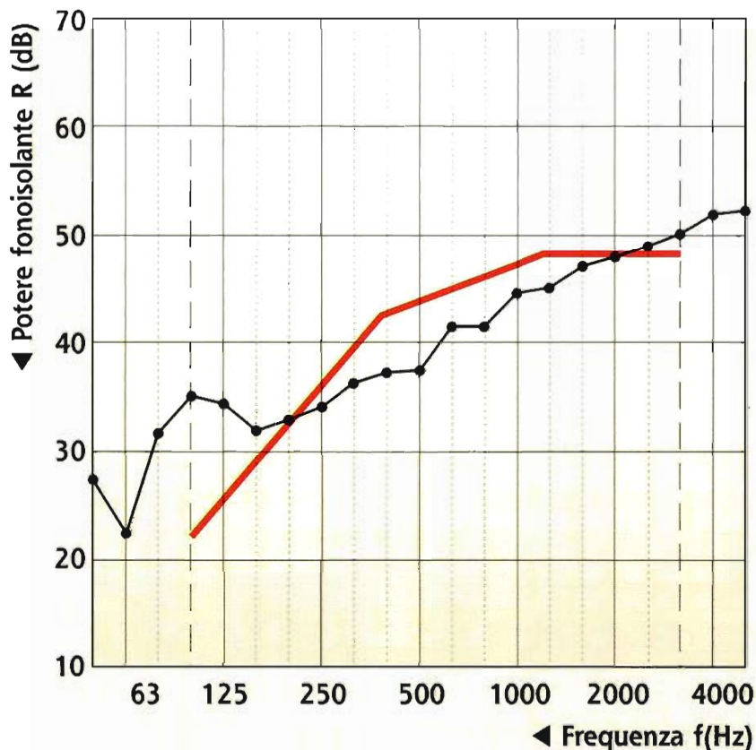
Fig. 23 - Il potere fonoisolante di una parete R (espresso in decibel, dB), verificato in laboratorio, viene documentato attraverso un certificato che riporta in un diagramma (—●—) la riduzione dell'energia sonora che si ha attraverso la parete alle diverse frequenze del suono (Hz). Per semplicità il diagramma viene confrontato con una spezzata (—) ad esso assimilabile e il potere fonoisolante della parete viene espresso attraverso l'indice di valutazione letto ( R_w ) sulla spezzata a 500 Hz. Nel caso in figura R_w = 44 dB.
