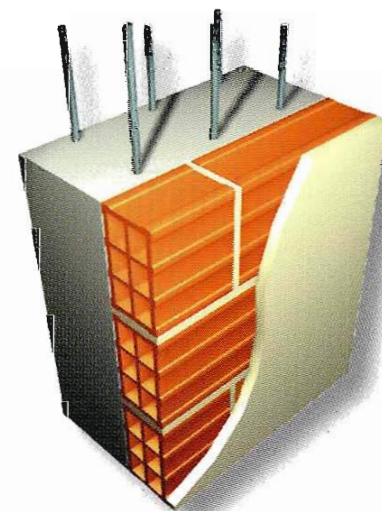
Fig. 5 - Controparete in elementi forati per murature portanti o setti in c.a.
